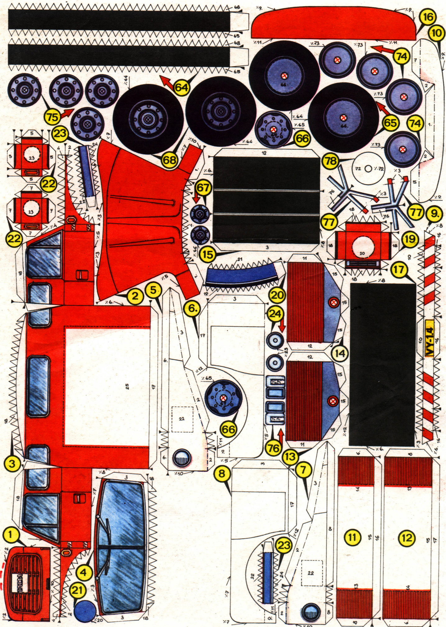
Vysokozdvíhací požární plošina PP 27
